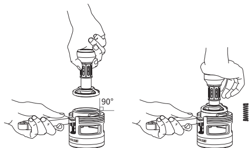
水平定圧、垂直タンピング
