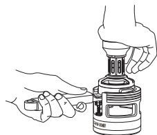
自適應高度 (填壓最高尺寸約13mm)
